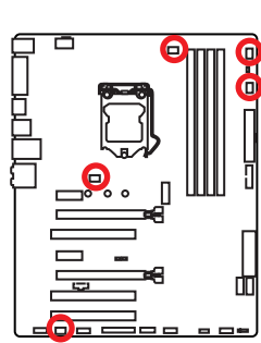
Разъем вентилятора с PWM управлением
