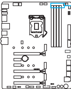
Indicateurs LED des barrettes DIMM
