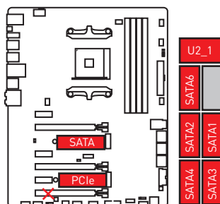
1xM.2 PCIe SSD + 1xM.2 SATA SSD + 5xSATA HDDs + 1xU.2 SSD
