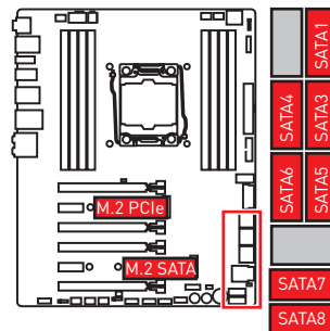
1xM.2 PCIe+ 1xM.2 SATA+ 7xSATA
