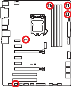
Connecteurs pour ventilateurs en mode PWM
